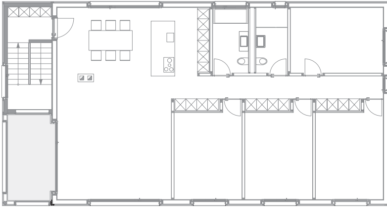
Grundriss Obergeschoss
