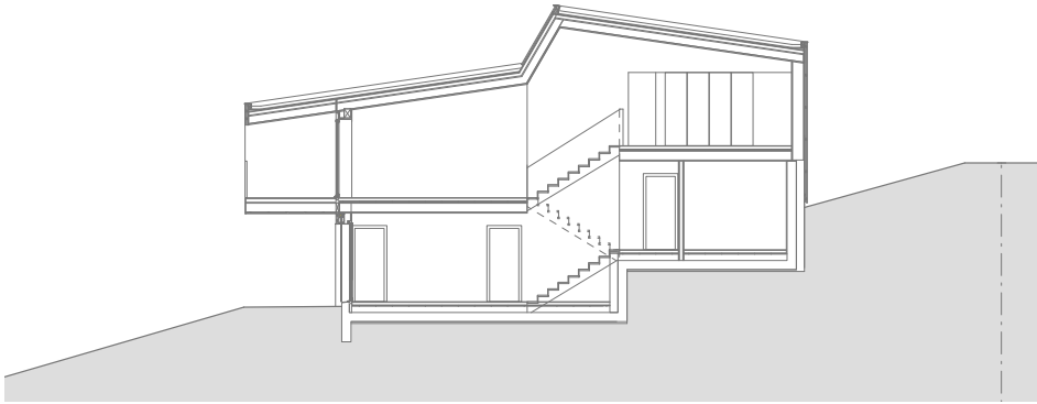
Schnitt
