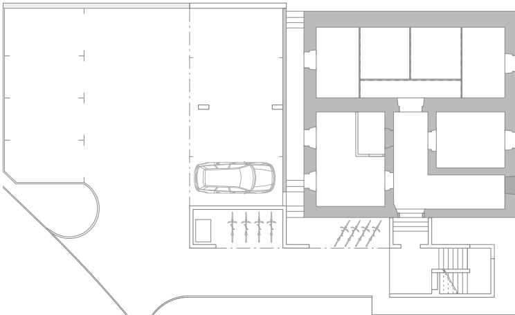
Grundriss Untergeschoss
