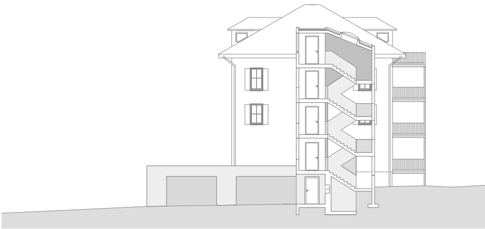
Schnitt
