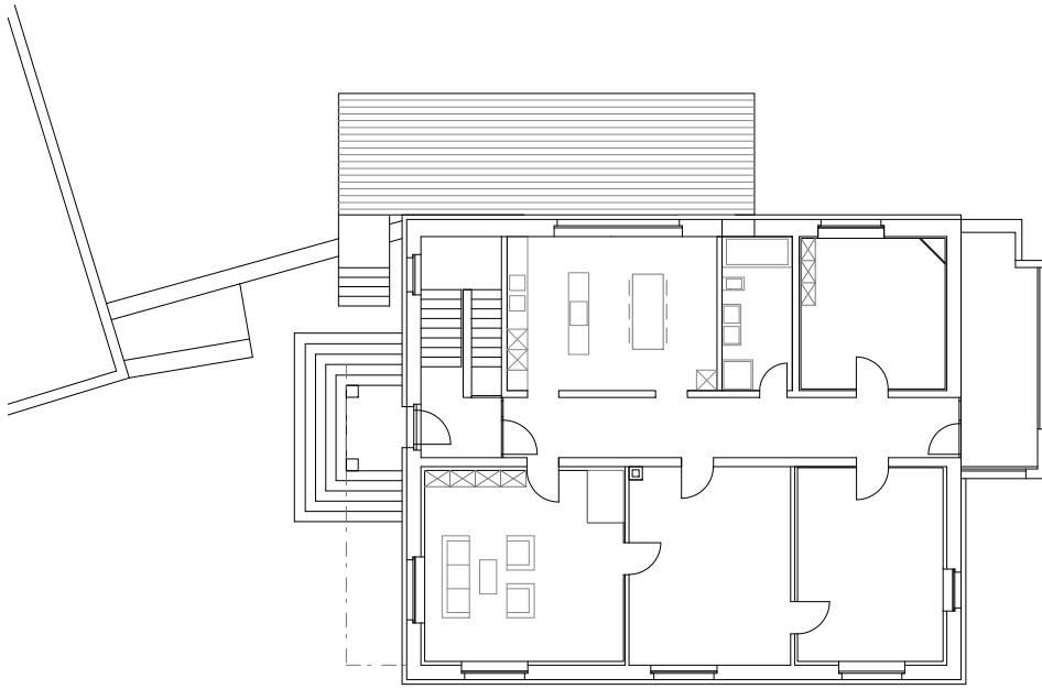
Grundriss Erdgeschoss
