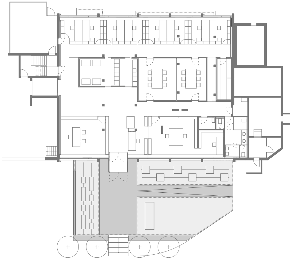
Grundriss Erdgeschoss
