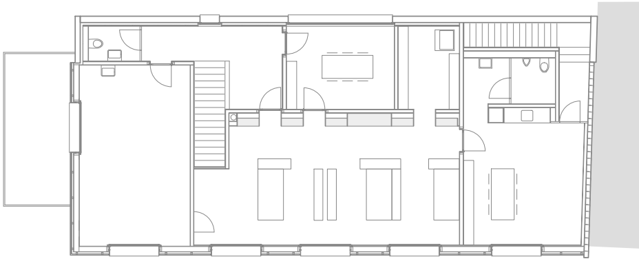
Obergeschoss
